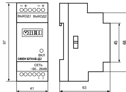
Рисунок 1 – Габаритные размеры блока
