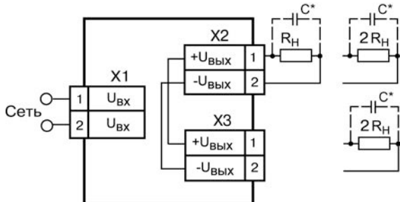
Рисунок 2 – Типовая схема подключения блока
