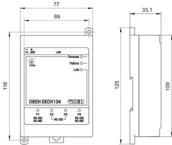
Рисунок А.1 – Габаритные и установочные размеры ОВЕН ЕКОН134
