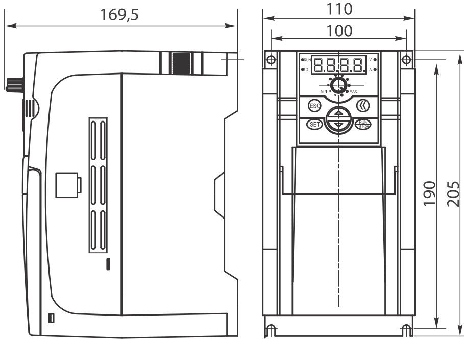
Габарит корпуса 3
