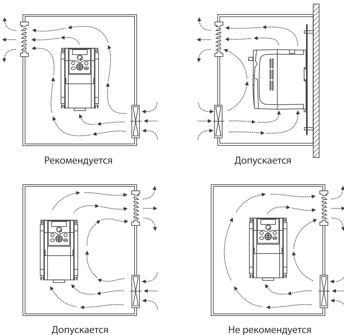
Рисунок 8 – Расположение элементов системы дополнительной вентиляции.
