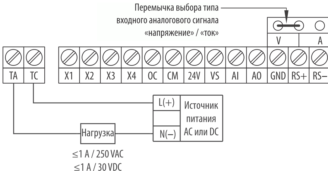
Рисунок 25 – схема подключения нагрузки к релейному выходу (питание от внешнего источника питания постоянного или переменного тока).
