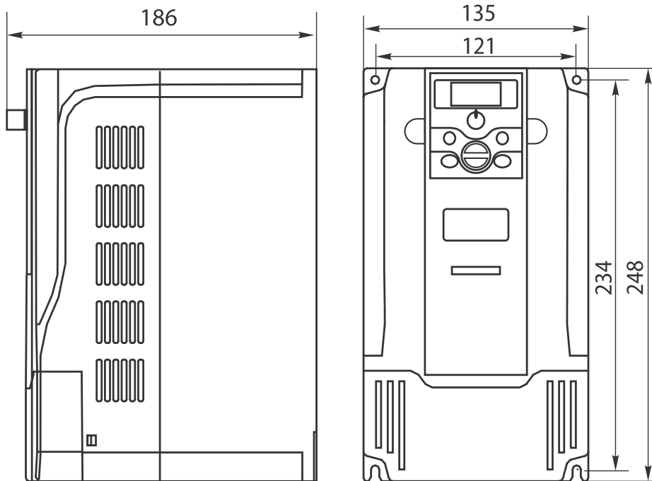
Габарит корпуса 4
