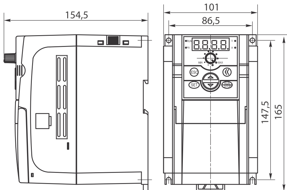
Габарит корпуса 2
