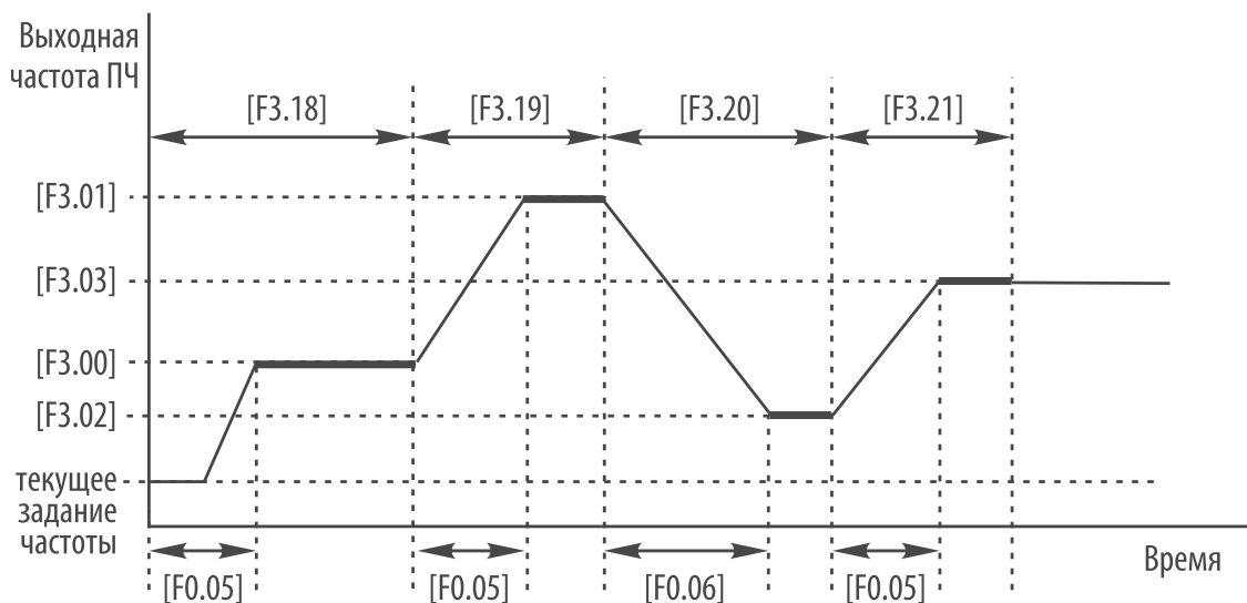
Рисунок 56 – режим программы ПЛК «Один цикл и работа на последней (четвертой) скорости».
