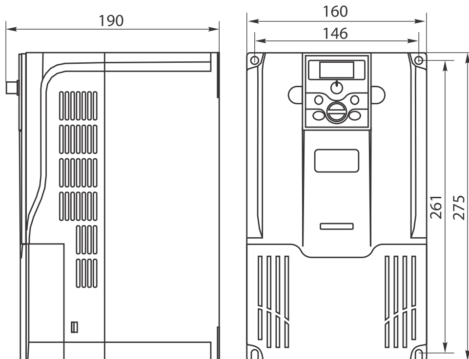
Габарит корпуса 5
