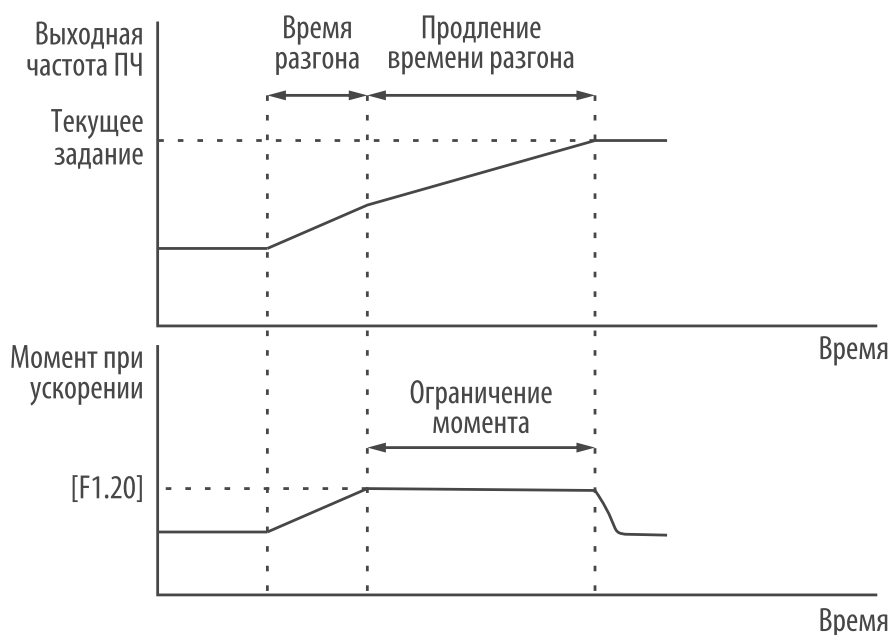
Рисунок 50 – ограничение момента при ускорении.
