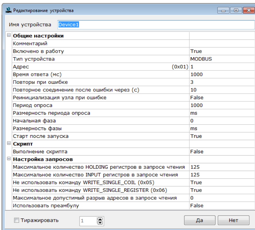
Рисунок 9.7 – Настройки устройства
