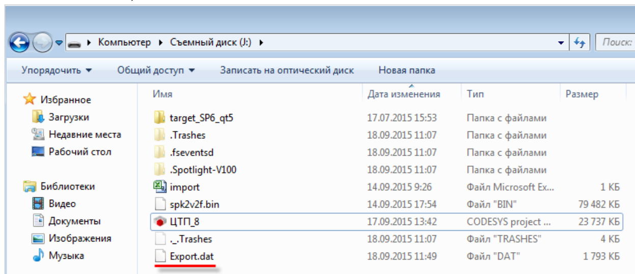
Рисунок 6.11 – Загрузка файла Export.dat в корень USB flash
