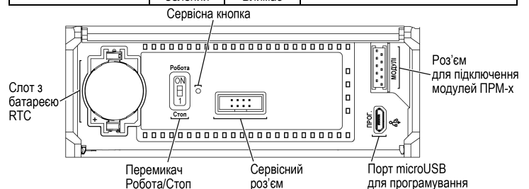
Рисунок 15 – Лицьова панель під кришкою
