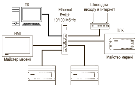
Рисунок 12 – Підключення за схемою «зірка»
