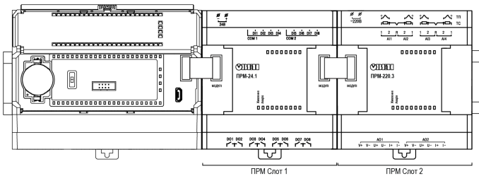
Рисунок 13 – Розташування модулів розширення на шині
