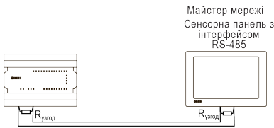
Рисунок 11 – Типова схема підключення у режимі Slave
