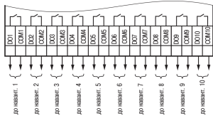
Рисунок 9 – Схема підключення навантажень до ВЕ типу «Р»
