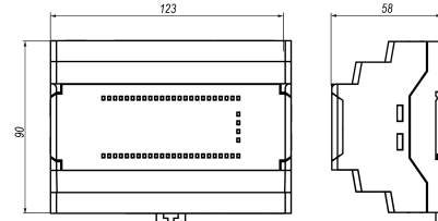
Рисунок 2 – Габаритні розміри пристрою
