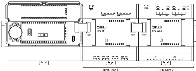
Рисунок 12 – Розташування модулів розширення на шині
