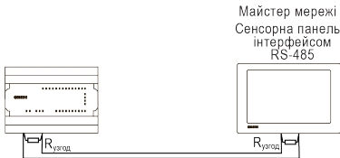
Рисунок 10 – Типова схема підключення у режимі Slave
