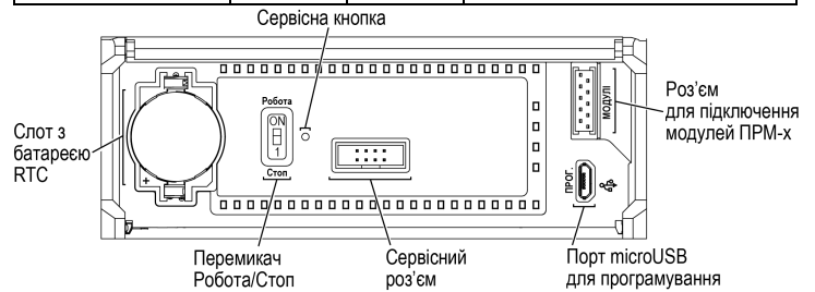
Рисунок 14 – Лицьова панель під кришкою
