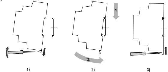
Рисунок 1 – Монтаж пристрою
