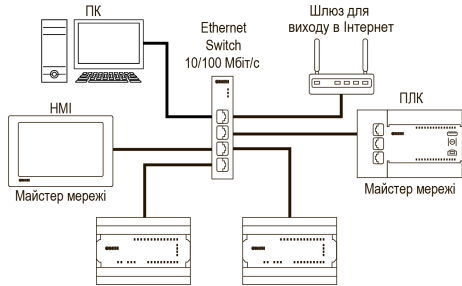
Рисунок 11 – Підключення за схемою «зірка»
