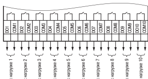
Рисунок 9 – Схема подключения нагрузок к ВЭ типа «Р»
