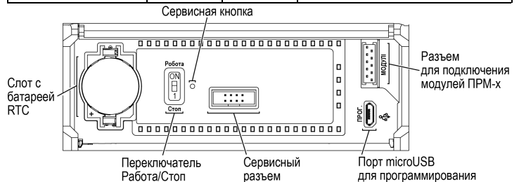
Рисунок 14 – Лицевая панель под крышкой
