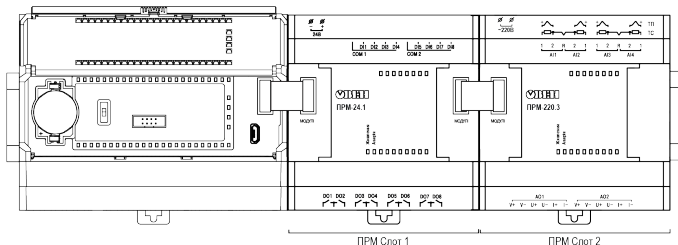
Рисунок 12 – Расположение модулей расширения на шине
