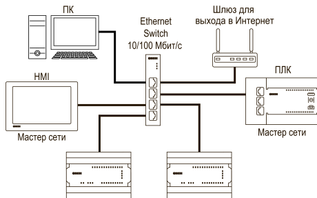
Рисунок 11 – Подключение по схеме «Звезда»
