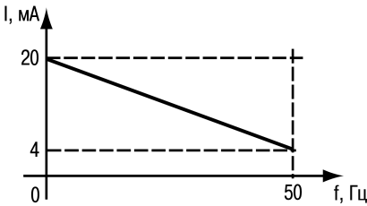
Рисунок 4.2 – Регулировочная характеристика ПЧВЗ
