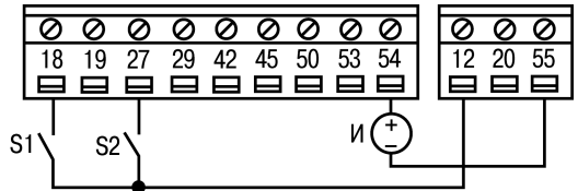
Рисунок 4.3 – Схема внешних подключений
