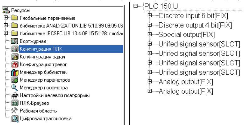
Рисунок 5.1 – Конфигурация ПЛК
