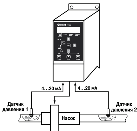
Рисунок 4.6 - Схема установки
