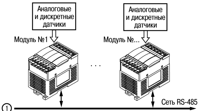
Рисунок 6.4 – Пример структуры соединений при использовании ПЛК в системе
