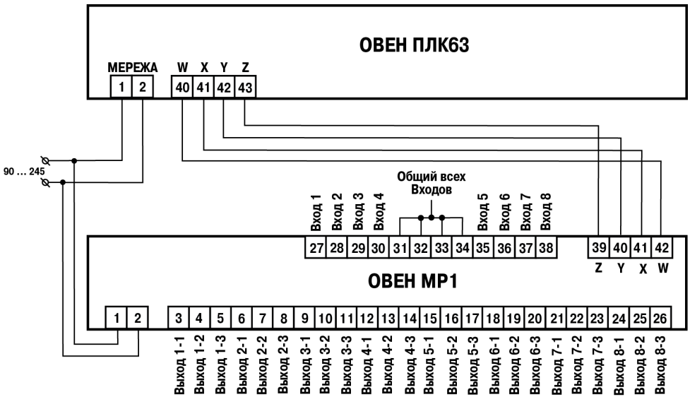
Рисунок Б.14 – Схема подключения модуля ОВЕН МР1 к контроллеру
