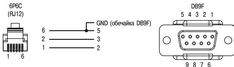
Рисунок В.2 – Схема кабеля программирования КС2
