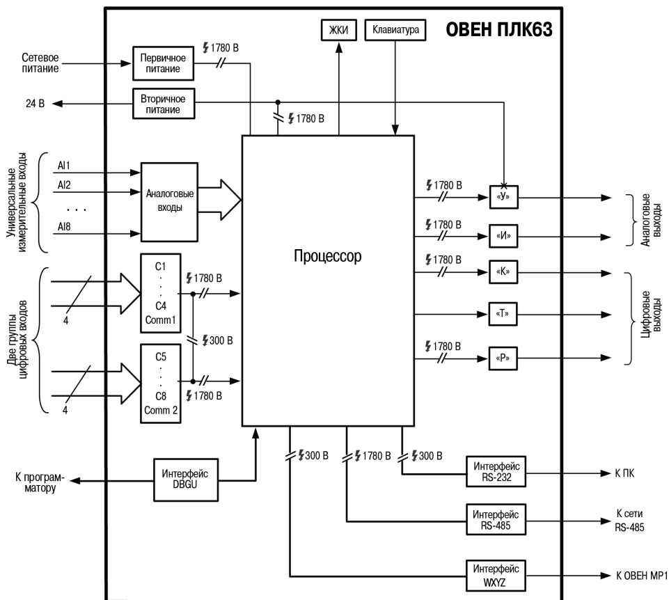
Рисунок 3.2 – Функциональная схема контроллера
