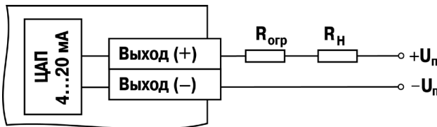
Рисунок 3.3 – Схема подключения нагрузки к ВУ типа «И»
