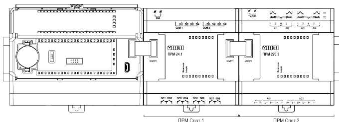
Рисунок 12 – Розташування модулів розширення на шині
