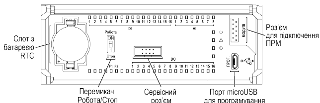
Рисунок 14 – Лицьова панель під кришкою
