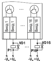
Рисунок 9 – Схема підключення навантажень до ВЕ типу «К»
