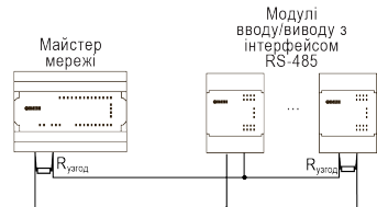
Рисунок 11 – Типова схема підключення у режимі Master
