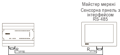
Рисунок 10 – Типова схема підключення у режимі Slave
