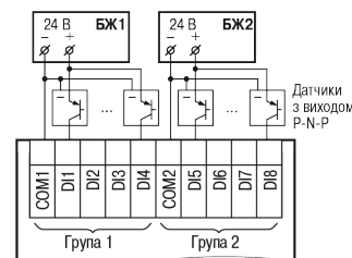
Рисунок 7 – Схема підключення до дискретних входів, що працюють у дискретному режимі, трипровідних дискретних датчиків, які мають вихідний транзистор п-р-п-типу з відкритим колектором для сигналів 24 В
