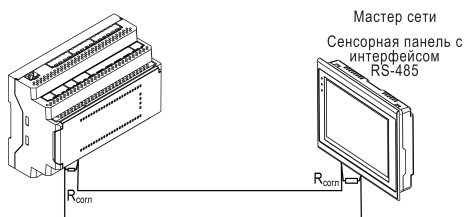
Рисунок 10 – Типовая схема подключения в режиме Slave
