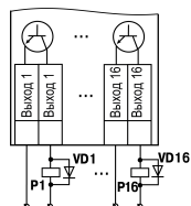
Рисунок 9 – Схема подключения нагрузок к ВЭ типа «К»
