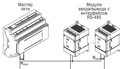
Рисунок 11 – Типовая схема подключения в режиме Master
