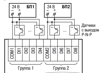
Рисунок 7 – Схема подключения к дискретным входам, работающим в дискретном режиме трехпроводных датчиков, имеющих выходной транзистор р-р-п-типа с открытым коллектором для сигналов 24 В
