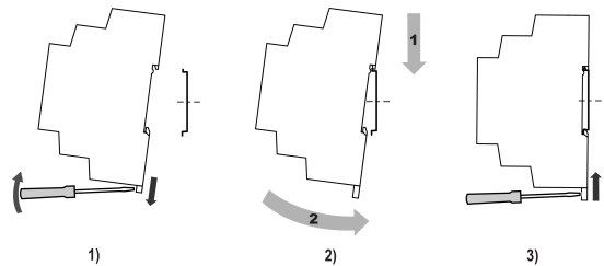
Рисунок 1 – Монтаж пристрою
