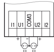
Рисунок 6 – Підключення датчиків з виходом у вигляді напруги
