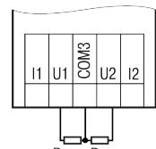
Рисунок 4 – Підключення резистивних датчиків
