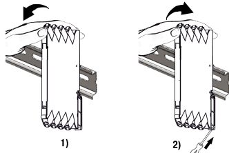
Рисунок 6.2 – Монтаж (1) і демонтаж (2) пристрою
