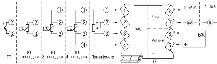
Рисунок 6.3 – Підключення пристрою
