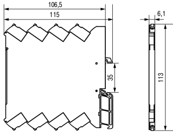
Рисунок 6.1 – Габаритний кресленник пристрою
