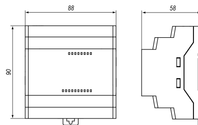
Рисунок 2 – Габаритні розміри
