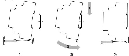
Рисунок 1 – Установлення пристрою
