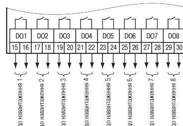
Рисунок 5 – Схема підключення навантаження до БЕ типу «Р»
