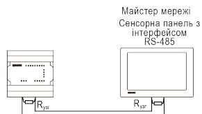
Рисунок 6 – Типова схема підключення для PR100 у режимі Slave
