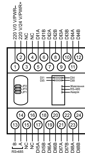
Рисунок 1 – Назначение контактов клеммника
