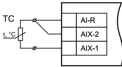
Рисунок 2 – Схема подключения термометра сопротивления
