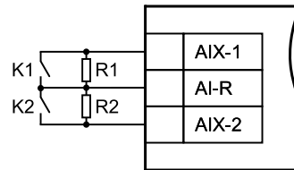
Рисунок 7 – Подключение «сухих контактов»
