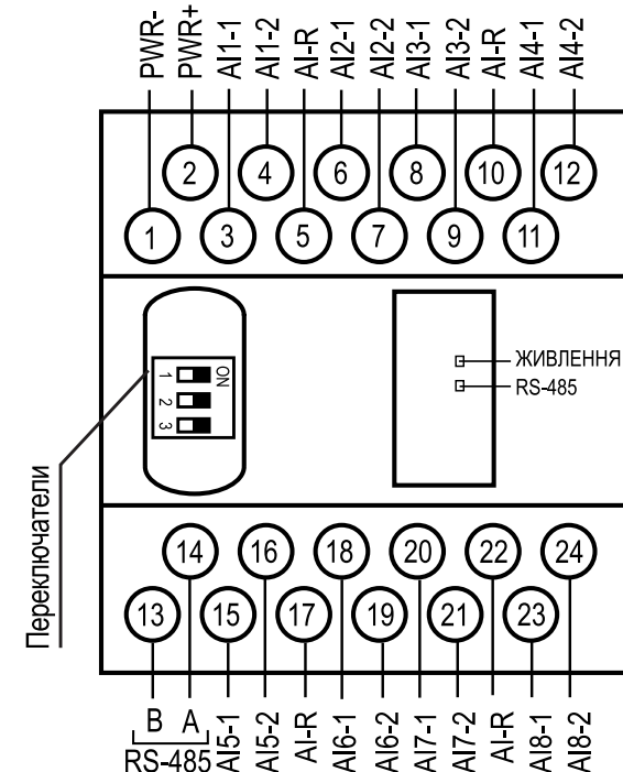
Рисунок 1 – Назначение контактов клеммника
