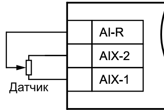
Рисунок 6 – Подключение резистивных датчиков положения
