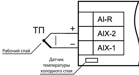
Рисунок 3 – Схема подключения термоэлектрического преобразователя
