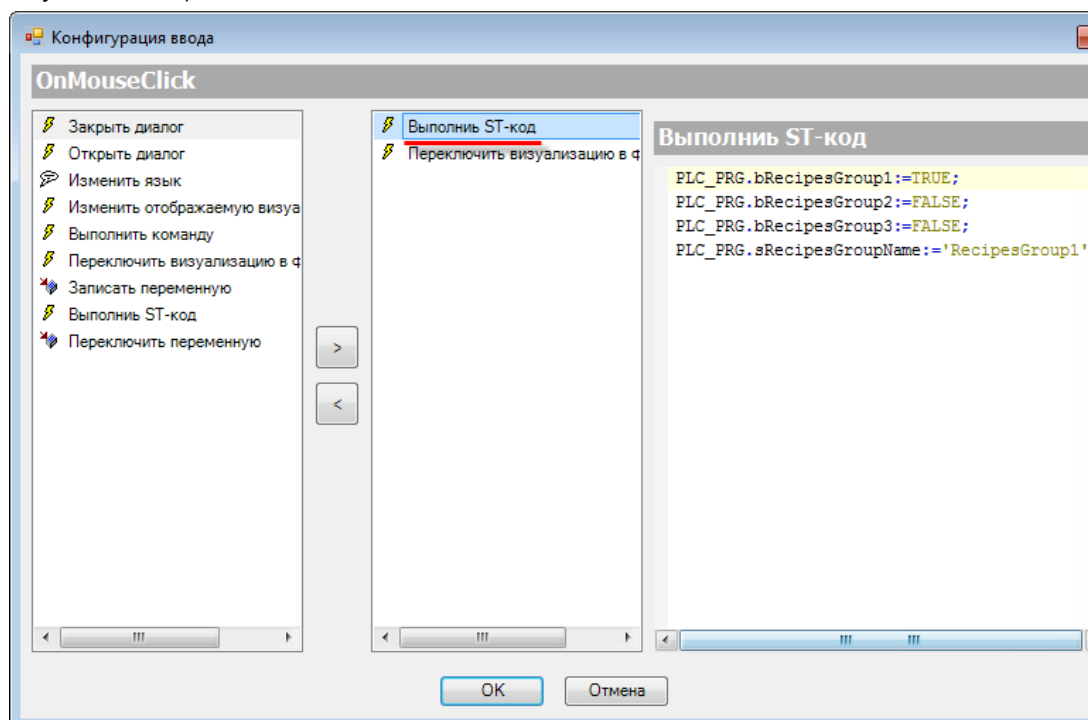
Рисунок 10.399 – Настройка параметра OnClick кнопки RecipesGroup1 , действие Выполнить ST-код
