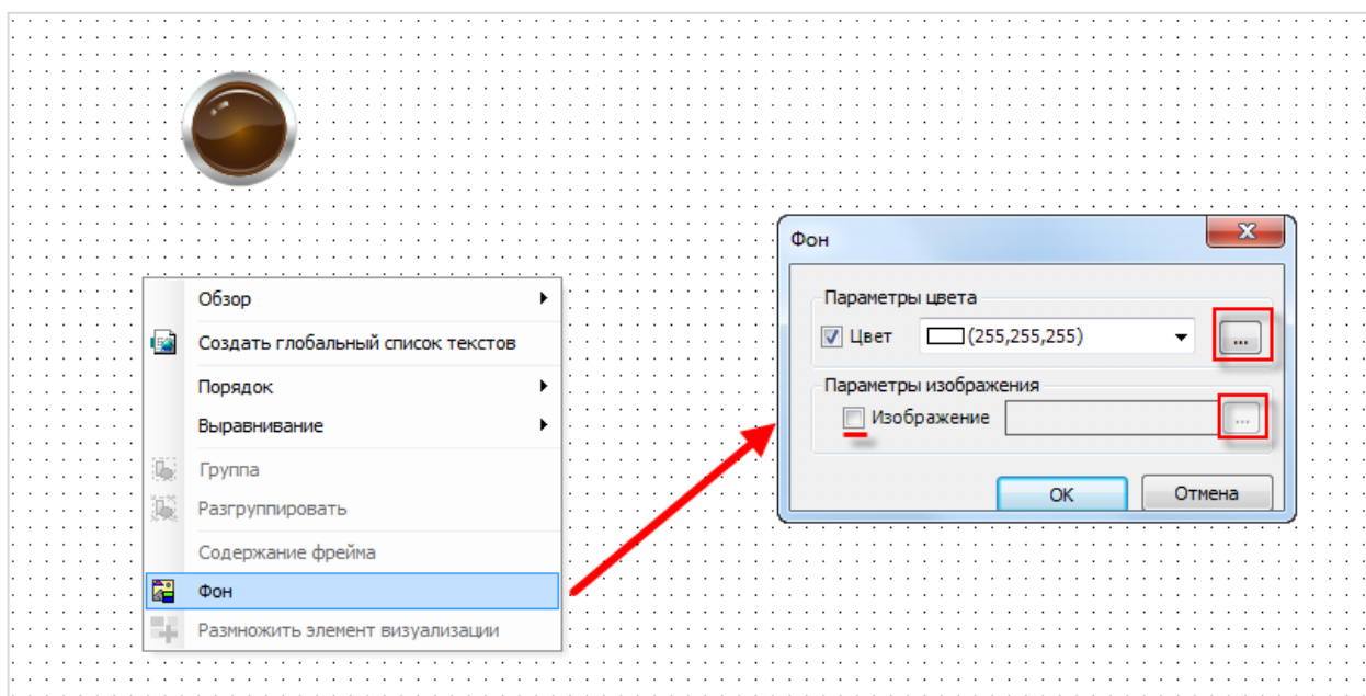
Рисунок 5.9 – Выбор фонового изображения экрана визуализации
