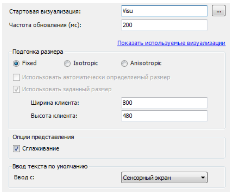
Рисунок 10.435 – Настройки таргет-визуализации
