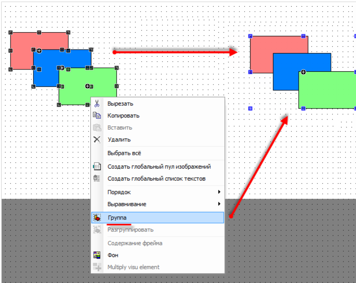
Рисунок 5.8 – Группировка элементов
