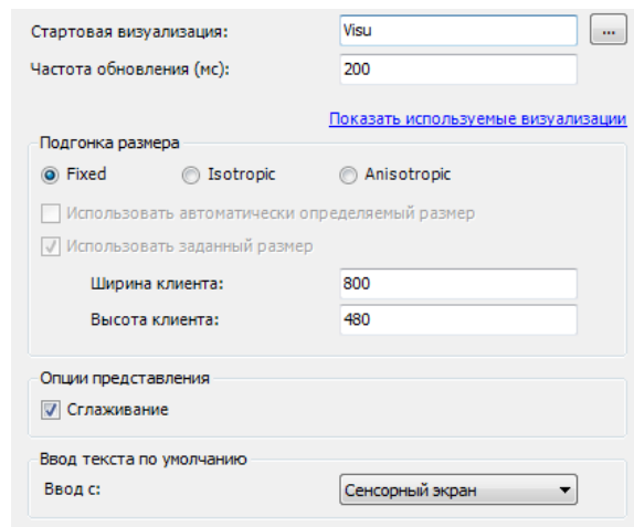
Рисунок 10.178 – Настройки таргет-визуализации
