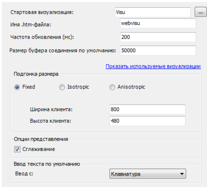
Рисунок 10.121 – Настройки web-визуализации
