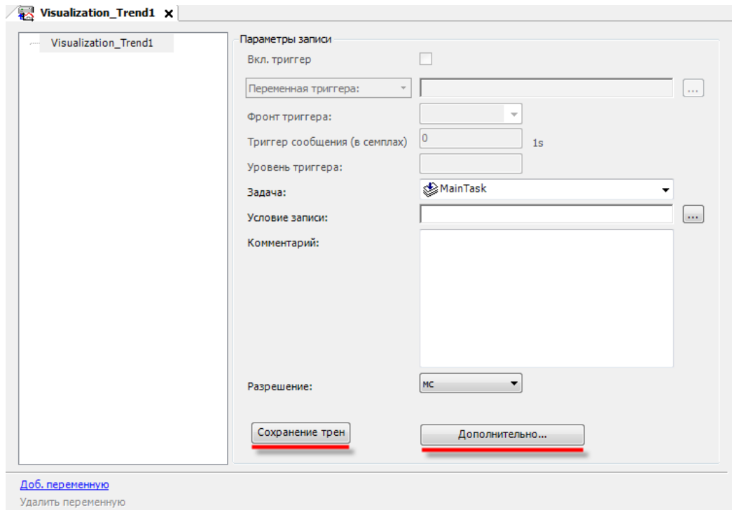
Рисунок 7.70 – Конфигурация тренда
