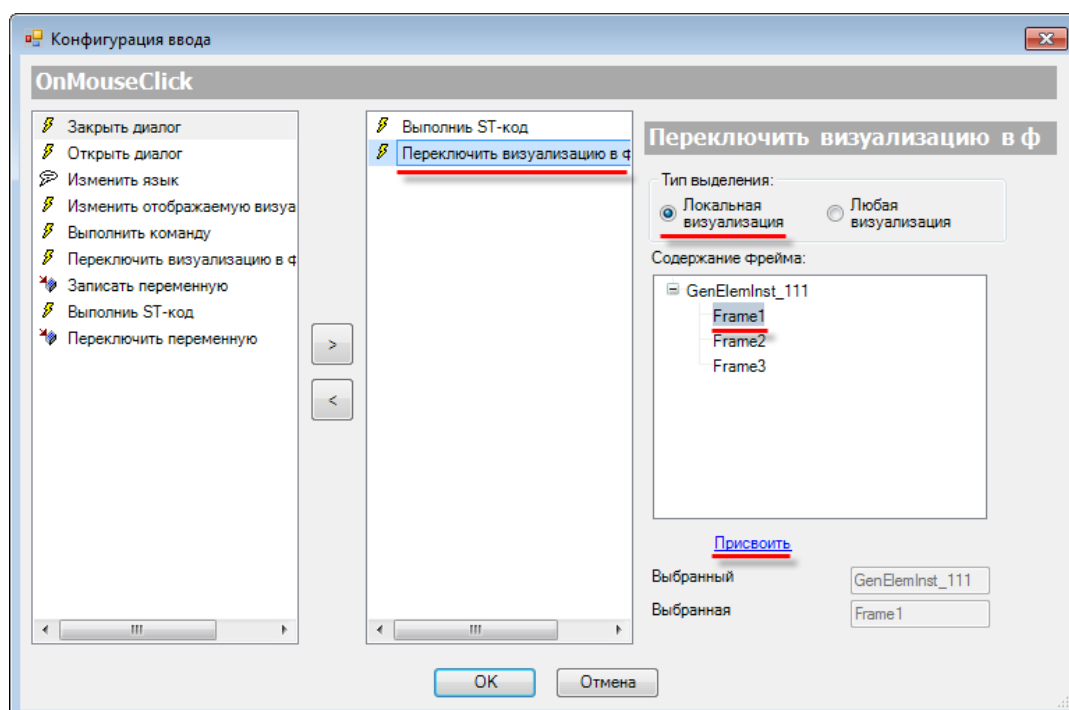
Рисунок 10.400 – Настройка параметра OnClick кнопки RecipesGroup1 , действие Переключить визуализацию во фрейме
