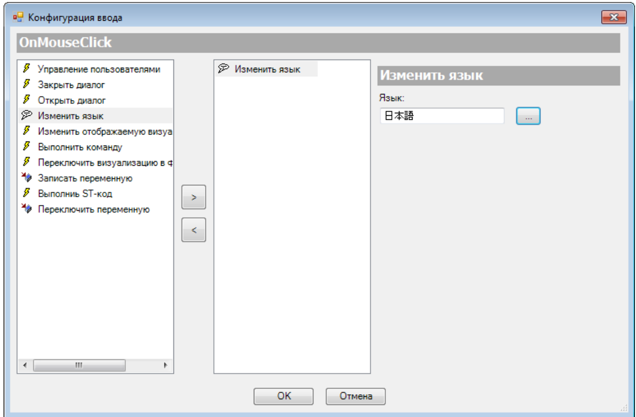
Рисунок 9.9 – Параметры действия Изменить язык
