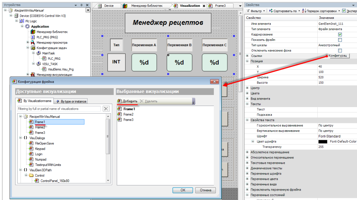
Рисунок 10.397 – Настройка содержимого элемента Фрейм
