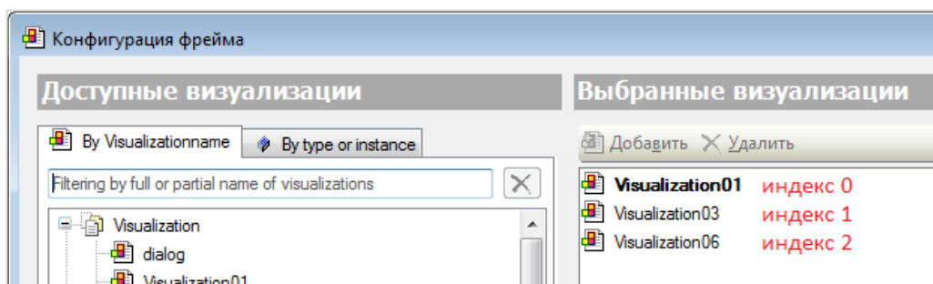
Рисунок 9.13 – Конфигурация фрейма
