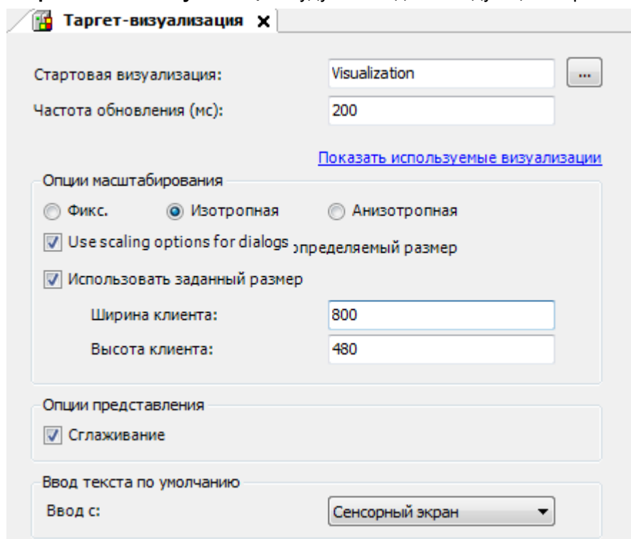
Рисунок 10.372 – Настройки таргет-визуализации
