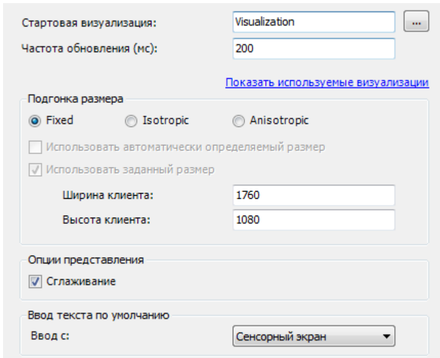
Рисунок 10.12 – Настройки таргет-визуализации
