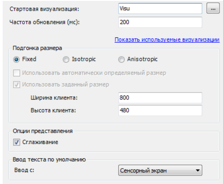
Рисунок 10.120 – Настройки таргет-визуализации
