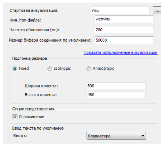
Рисунок 10.179 – Настройки web-визуализации
