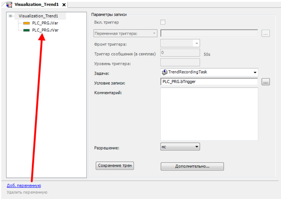
Рисунок 10.165 – Конфигурация тренда
