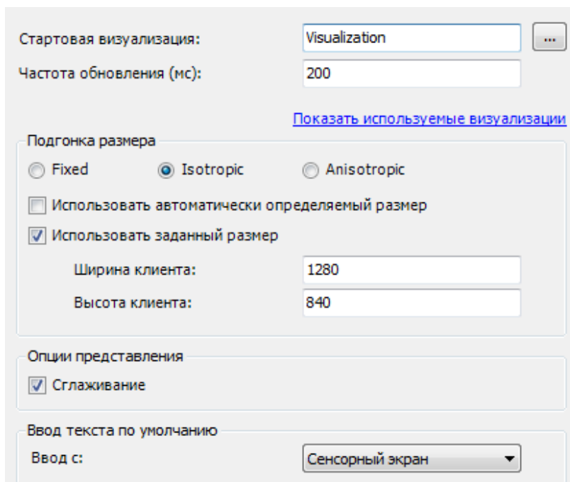
Рисунок 10.233 – Настройки таргет-визуализации
