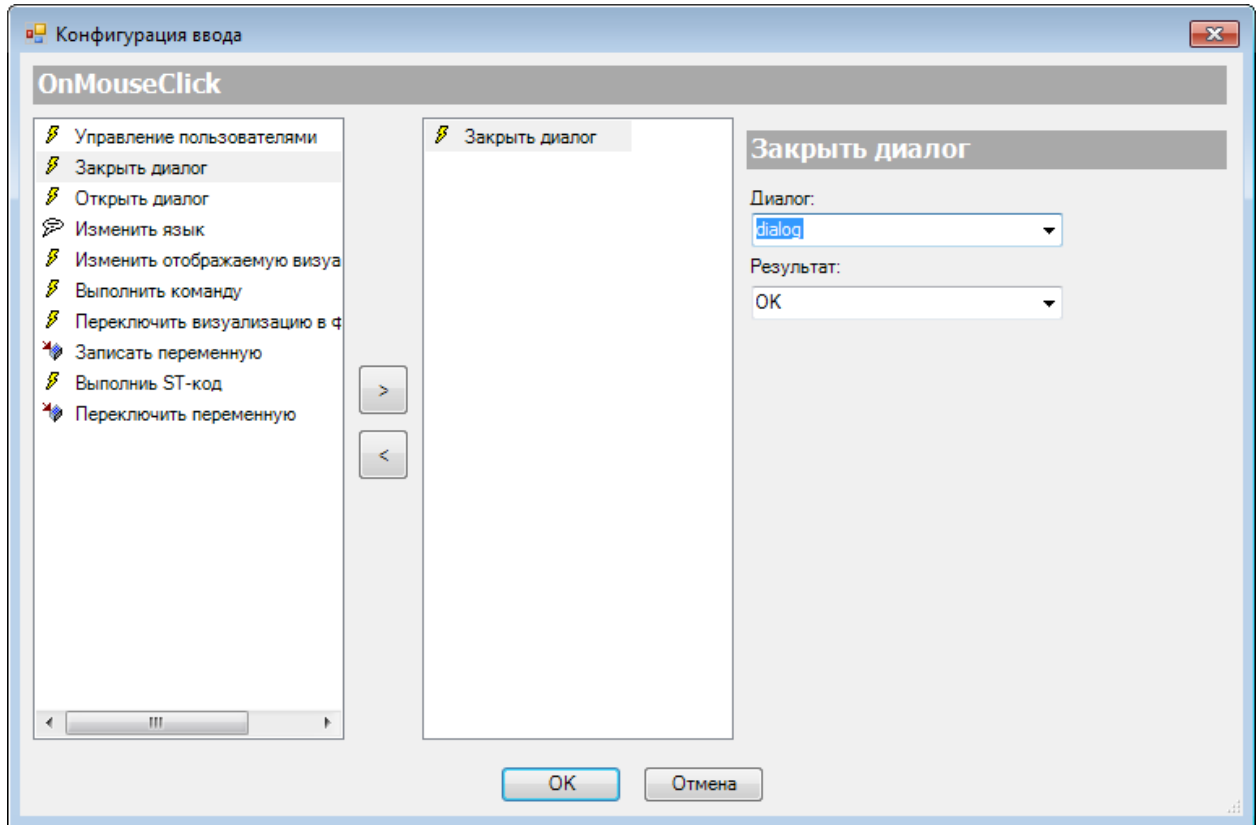
Рисунок 9.7 – Параметры действия Закреть диалог
