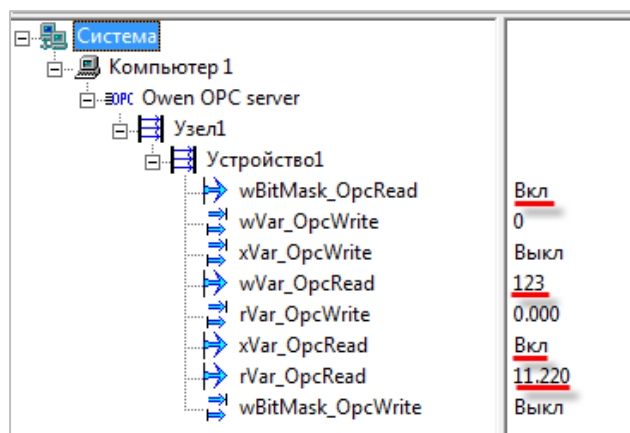
Рисунок 4.7.6 – Считывание данных из контроллера в MasterSCADA
