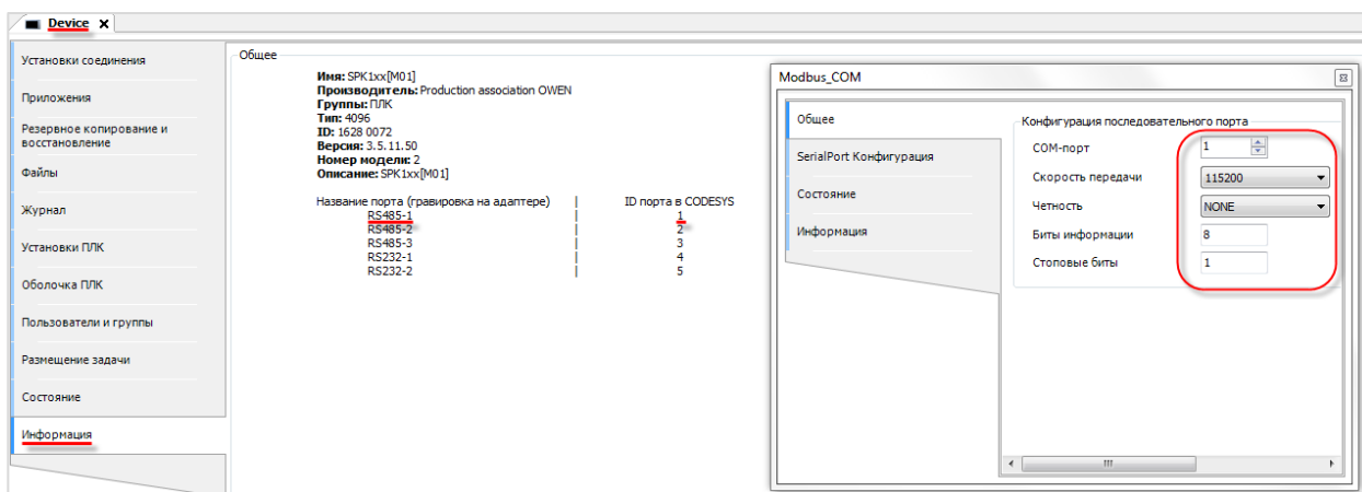
Рисунок 7.144 – Настройки компонента Modbus COM
