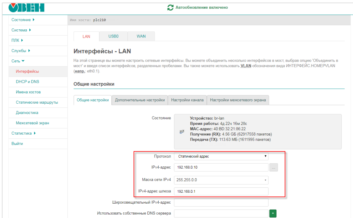
Рисунок 5.3 – Сетевые настройки интерфейса
