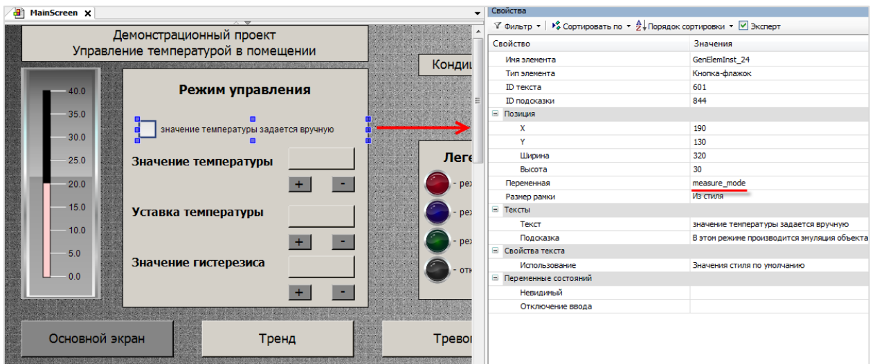
Рисунок 7.108 – Привязка переменной measure_mode к чекбксу
