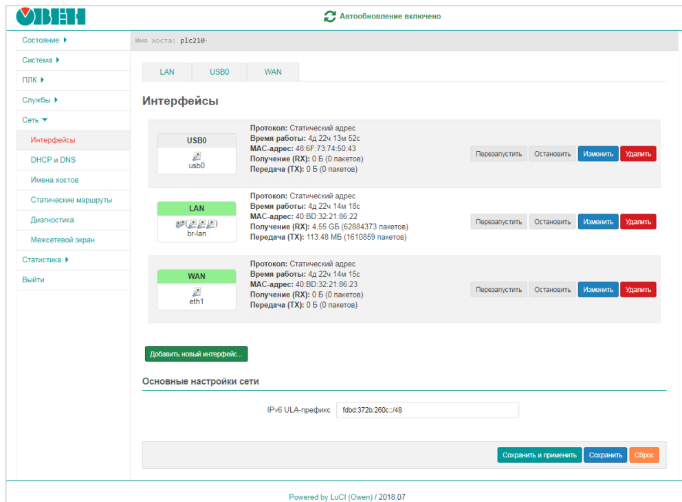
Рисунок 5.2 – Список интерфейсов контроллера
