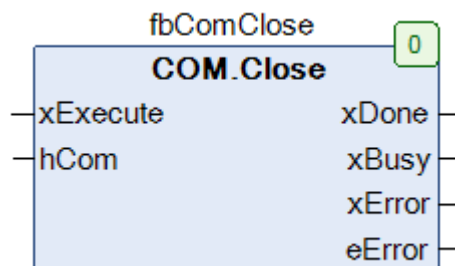
Рисунок 3.5 – Внешний вид ФБ COM.Close на языке CFC
