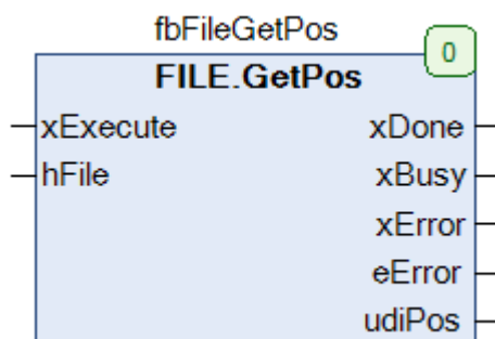
Рисунок 4.17 – Внешний вид ФБ FILE.GetPos на языке CFC
