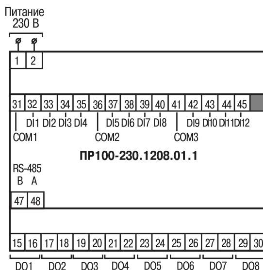
Рисунок А.4 – Расположение контактов для PR100-230.1208.01.1
