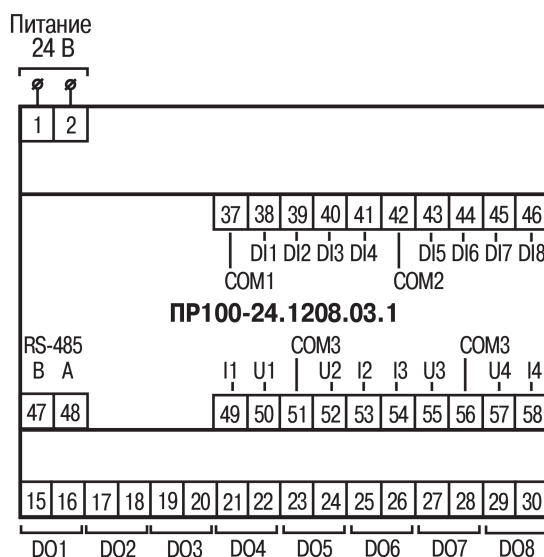
Рисунок А.2 – Расположение контактов для PR100-24.1208.03.1
