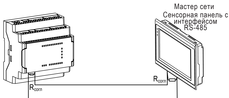
Рисунок 5.7 – Типовая схема подключения для ПР100 в режиме Slave
