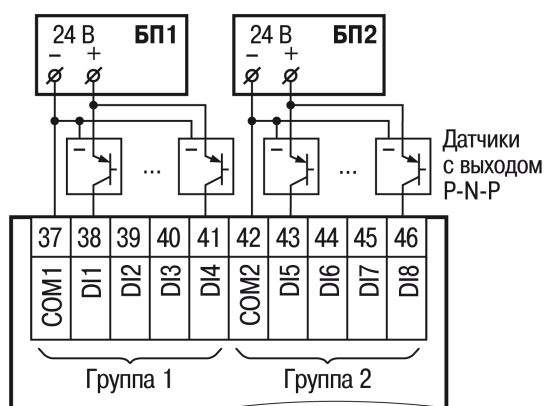
Рисунок 5.3 – Схема подключения датчиков с выходным транзистором р-п-п типа к входам типа «Д»
