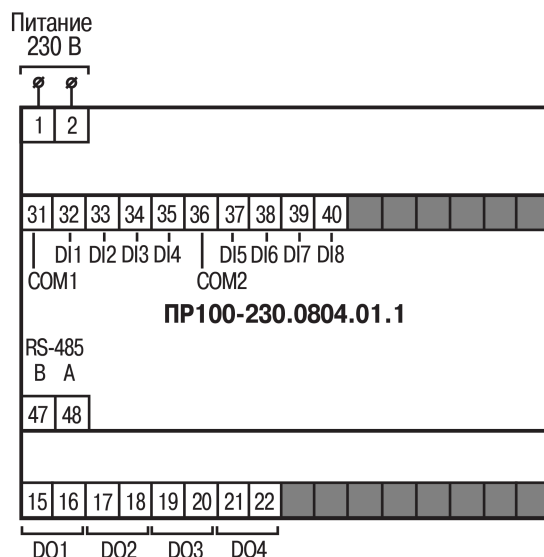
Рисунок А.3 – Расположение контактов для PR100-230.0804.01.1
