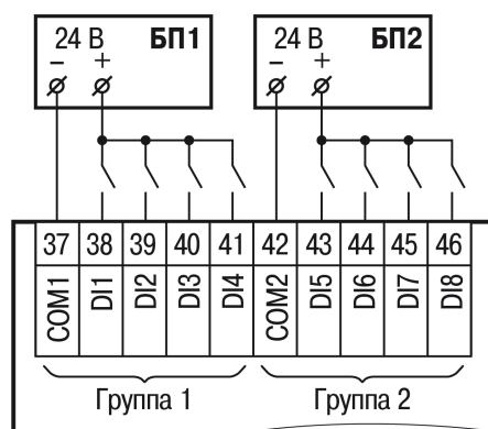
Рисунок 5.2 – Схема подключения дискретных датчиков с питанием 24 В к входам типа «Д»
