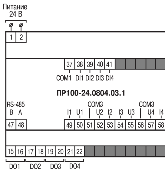
Рисунок А.1 – Расположение контактов для ПР100-24.0804.03.1
