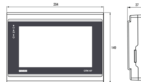
Рисунок 1 – Габаритные размеры прибора
