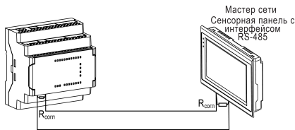
Рисунок 9 – Типовая схема подключения для PR100 в режиме Slave
