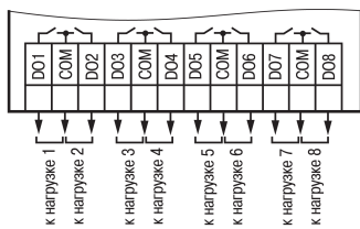
Рисунок 8 – Подключение нагрузки к ВЭ типа «Р»
