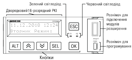
Рисунок 10 – Лицьова панель пристрою (кришку відсіку підключення модулів умовно не показано)
