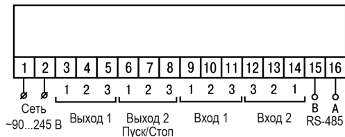
Рисунок 5.2 – Общая схема подключения TRM210-N, -Щ1 и -Щ2
