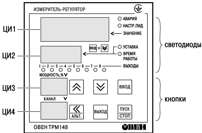
Рисунок 4.1 – Лицевая панель прибора
