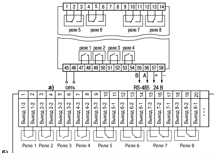
Рисунок Б.2 – Схема подключения электромагнитных реле прибора TRM148-Р: а) в корпусе Щ4, б) в корпусе Щ7
