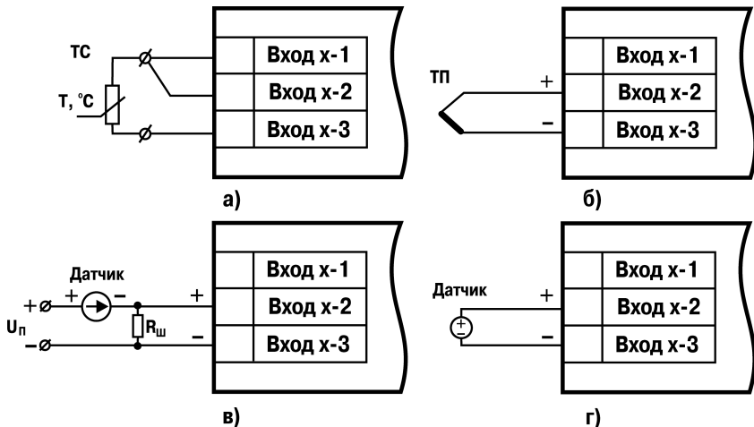
Рисунок Б.9 – Схемы подключения измерительных датчиков: а) термопреобразователи сопротивления; б) термопары; в) датчик с выходным сигналом тока от 0 (4) до 20 мА, от 0 до 5 мА ( R_{ш}=50,000 \pm 0,025 \text{ Ом} ); г) датчик с выходным сигналом напряжения от 0 до 50 мВ, от 0 до 1 В
