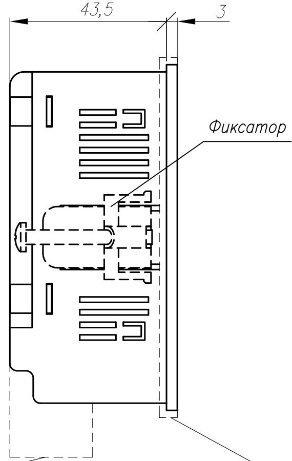
Вид слева
