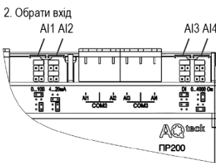
Рисунок 3 – Схема налаштування А1...А4
