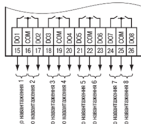
Рисунок 7 – Підключення навантаження до ВЕ типу «Р»
