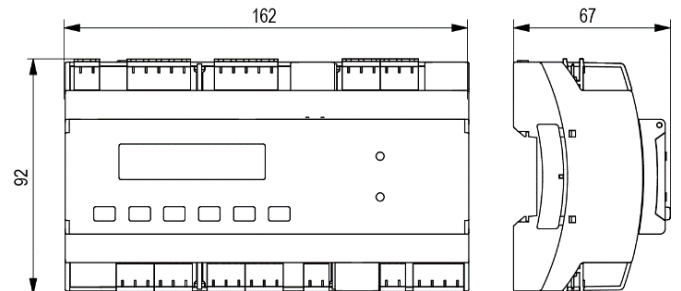
Рисунок 2 – Габаритний креслення пристрою
