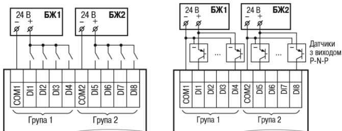
Рисунок 5 – Підключення дискретних датчиків з живленням 24 В
