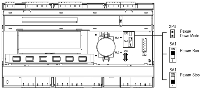
Рисунок 4 – Вид на верхню плату з відкритою кришкою
