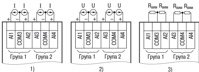
Рисунок 6 – Підключення: 1) активних датчиків з виходом типу «Струм 4...20 мА», 2) активних датчиків з виходом типу «Напруга 0...10 мА», 3) датчиків опору з діапазоном 0...4000 Ом
