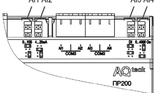
Рисунок 3 – Схема налаштування A11...A14
