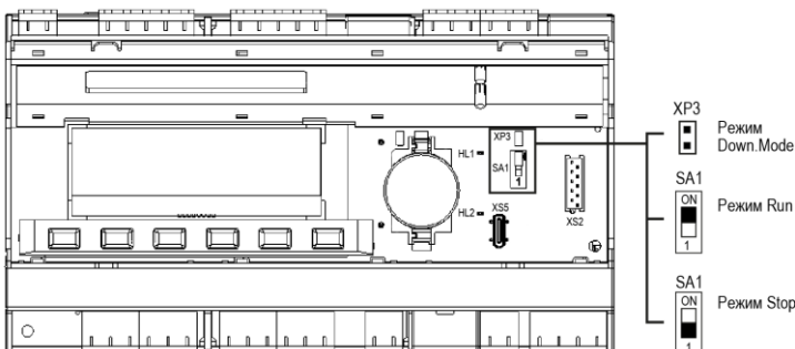
Рисунок 4 – Вид на верхню плату з відкритою кришкою
