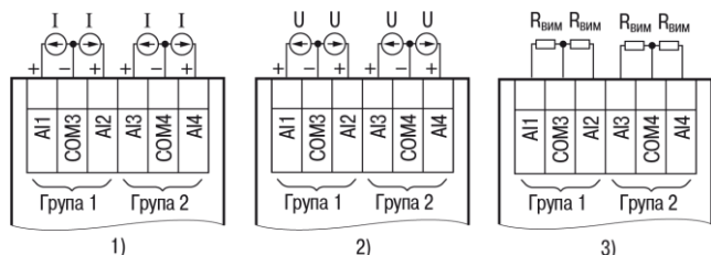
Рисунок 6 – Підключення: 1) активних датчиків з виходом типу «Струм 4...20 мА», 2) активних датчиків з виходом типу «Напруга 0...10 мА», 3) датчиків опору з діапазоном 0...4000 Ом
