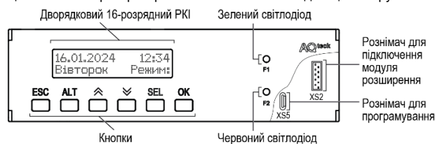
Рисунок 9 – Лицьова панель пристрою
