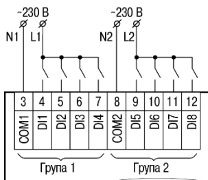
Рисунок 5 – Підключення дискретних датчиків з живленням 230 В
