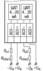
Рисунок 8 – Підключення навантаження до ВЕ типу «И»
