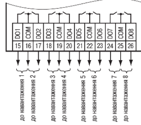
Рисунок 7 – Підключення навантаження до ВЕ типу «Р»
