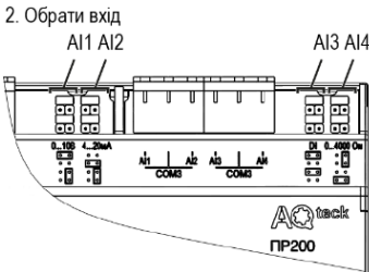
Рисунок 3 – Схема налаштування AI1...AI4
