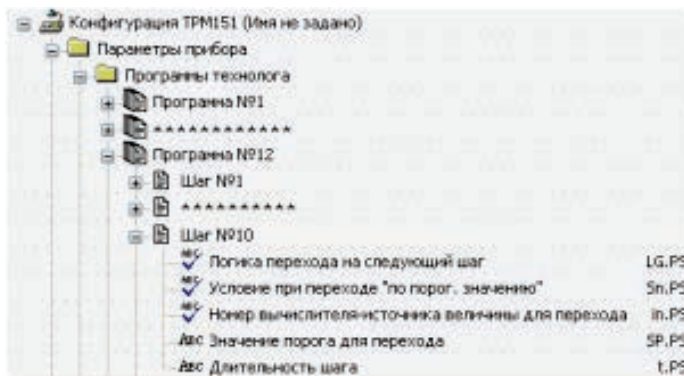
Рисунок 3.3 – Примеры Программ, реализуемых с применением различных видов шагов
