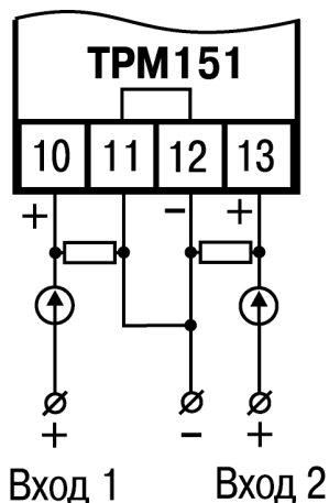
Рисунок 8.10 – Схема подключения активных датчиков типа «параметр-ток», «параметр-напряжение»
