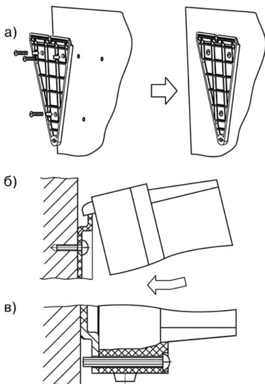
Рисунок 8.1 – Установка прибора настенного крепления
