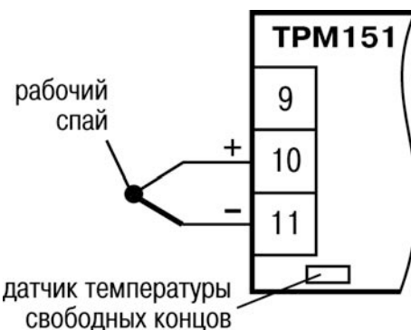
Рисунок Г.2 – Подключение термопары
