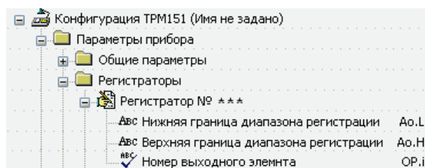
Рисунок 3.24 – Работа Регистратора
