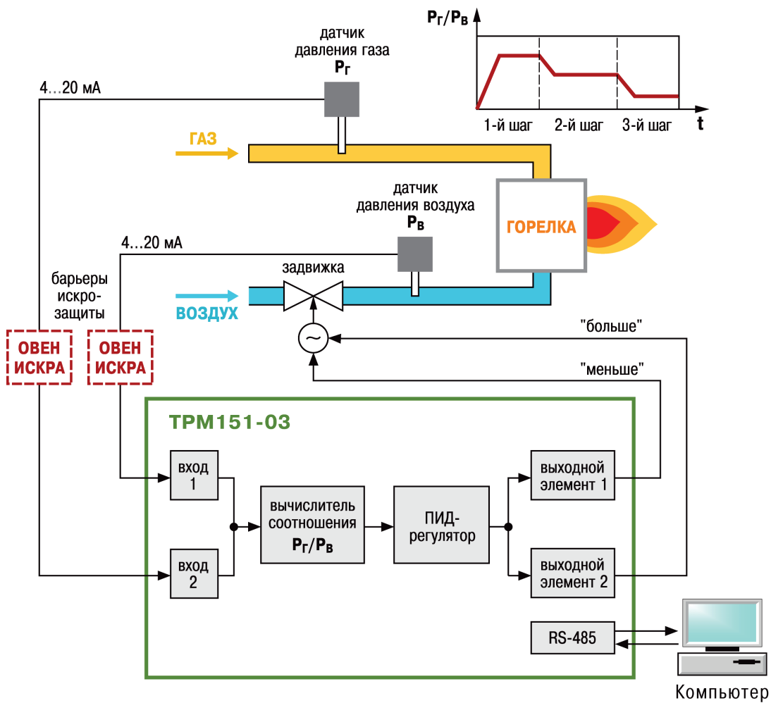
Рисунок 4.4 – Использование канального регулятора TRM151 03й модификации в качестве регулятора соотношения газ/воздух
