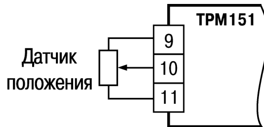
Рисунок 8.11 – Схема подключения резистивного датчика
