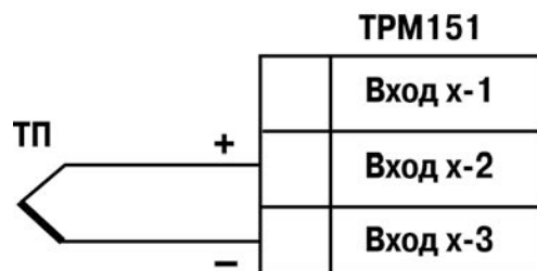
Рисунок Б.5 – Схема подключения преобразователя термоэлектрического
