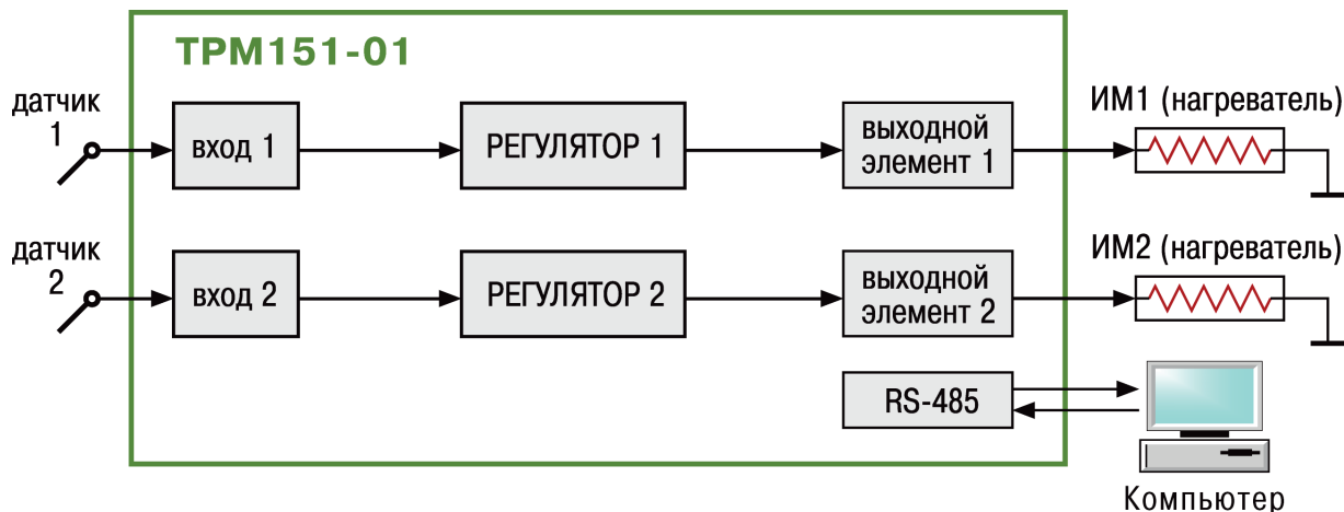
Рисунок 4.1 – Принципиальная схема модификации 01 прибора ТРМ151
