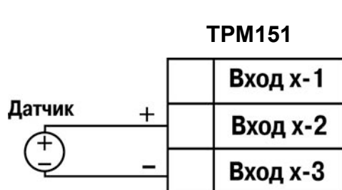
Рисунок Б.6 – Схема подключения активного датчика с выходом в виде напряжения 0...50 мВ или 0...1 В
