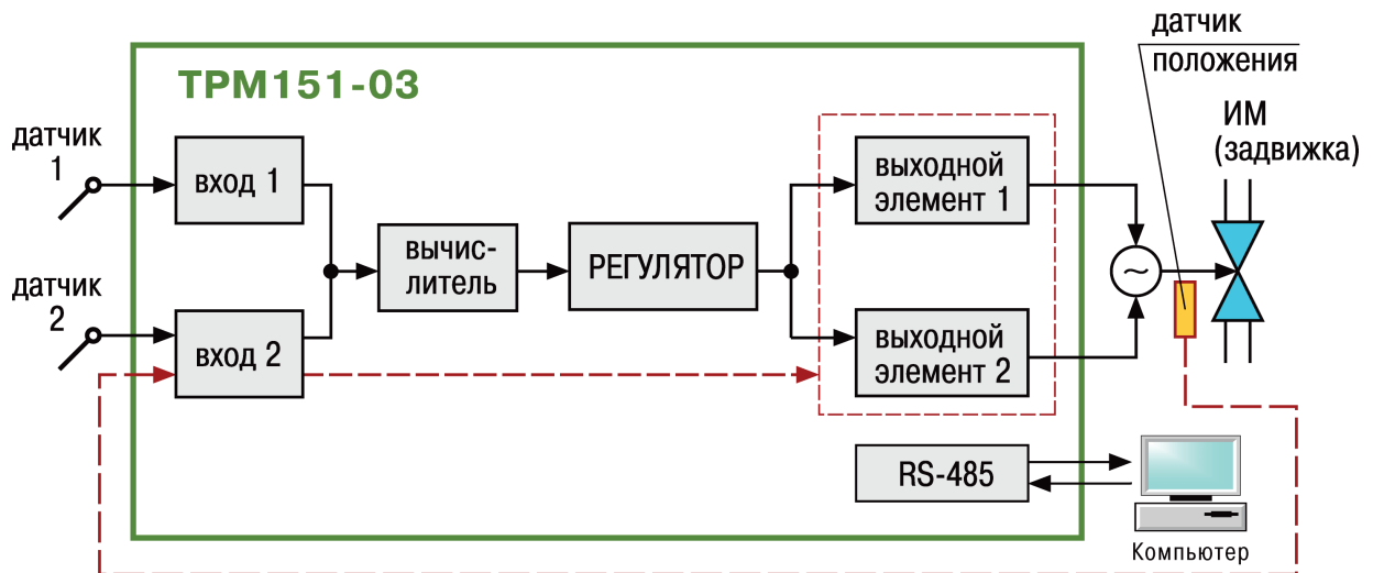
Рисунок 4.3 – Принципиальная схема модификации 03 прибора ТРМ151
