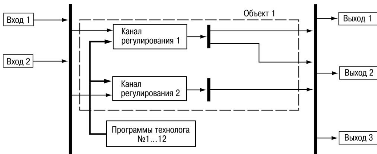
Рисунок 3.1 – Структурная схема прибора TPM151
