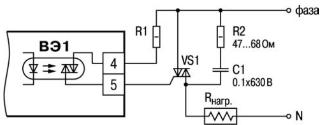
Рисунок 8.4 – Схема подключения нагрузки к ВЭ типа «Оптосимистор»
