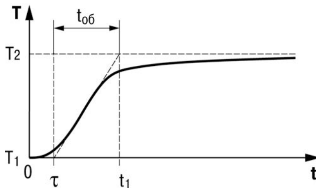
Рисунок Ж.3 – График переходной функции
