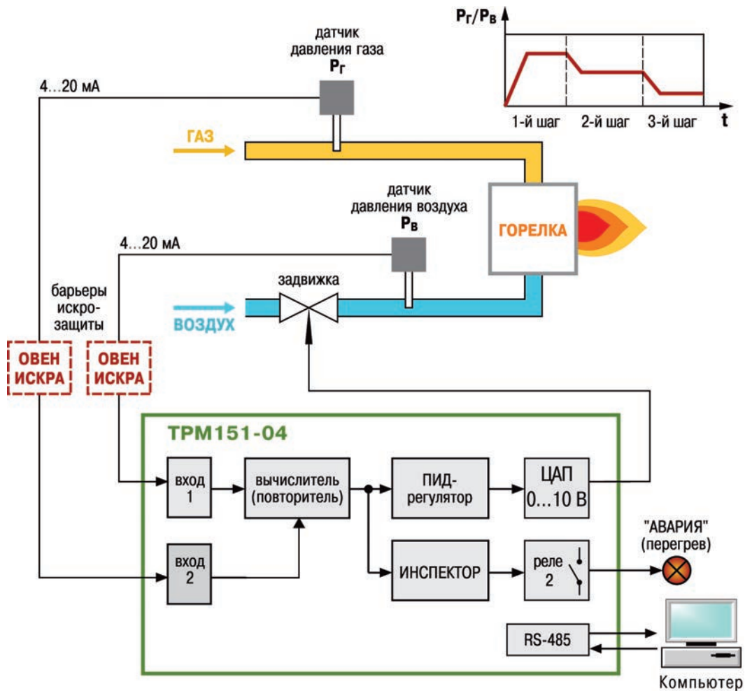
Рисунок 4.7 – Использование 1-канального регулятора TRM151 04й модификации в качестве регулятора соотношения газ/воздух
