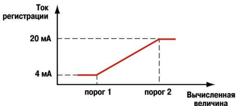
Рисунок 3.24 – Работа Регистратора
