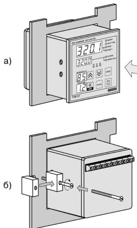
Рисунок 8.2 – Установка прибора щитового крепления
